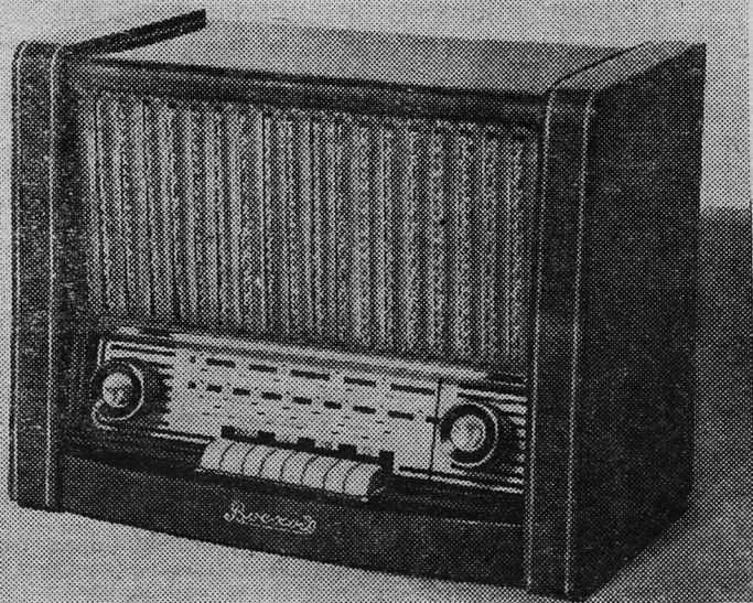
Ленинград. Радиоприемник «Восход» супергетеродинного типа предназначен для сельской местности, где отсутствует электрическая сеть. На Всемирной выставке в Брюсселе этот приемник в комплексе приемников «Спутник» и «Сюрприз» удостоен Золотой медали.
