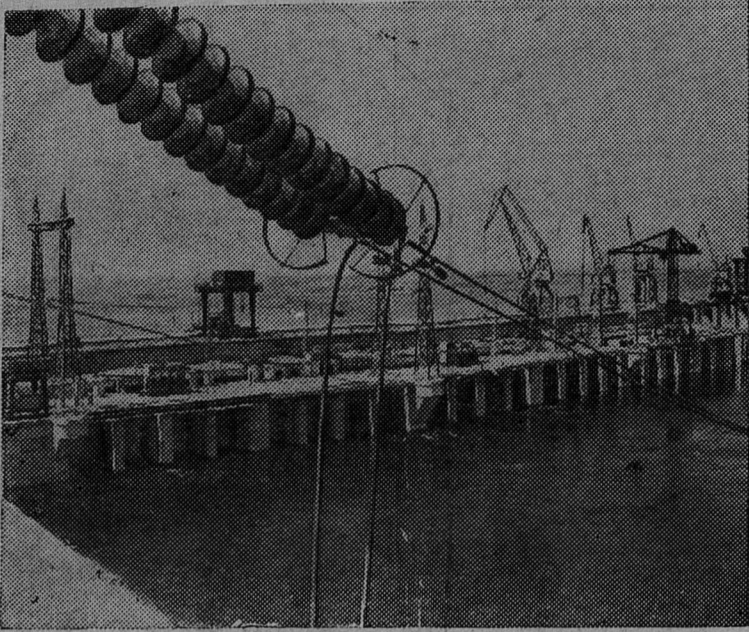
УКРАИНСКАЯ ССР. Строительство Кременчугской ГЭС подходит к концу. Ныне действующие 7 агрегатов этой мощной электростанции на Днепре выработали более 200 миллионов киловатт-часов электроэнергии. Остальные 5 агрегатов
