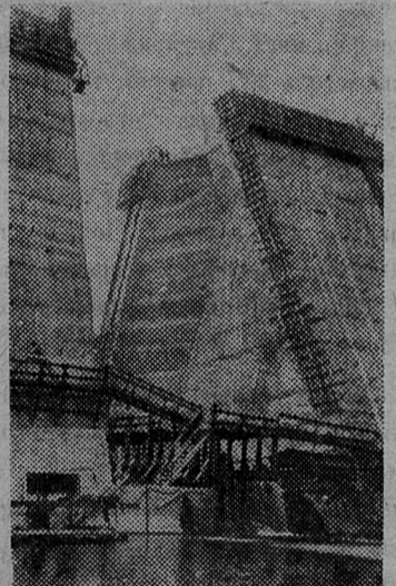
ЧЕХОСЛОВАЦКАЯ РЕСПУБЛИКА. Строительство Флайской плотины. Она будет состоять из 35 блоков. Ее высота достигнет 50 метров. Чехословацкое телеграфное агентство.
