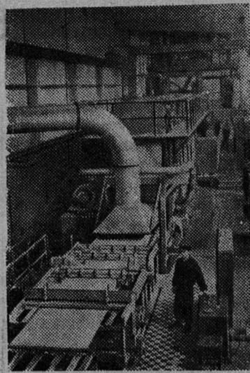
ЛЕНИНГРАД. На Дубровском домостроительном комбинате закончен монтаж нового цеха-автомата по производству древесностружечных плит. Мощность оборудования рассчитана на получение в среднем двух миллионов квадратных метров этих изделий в год. Весь технологический процесс автоматизирован. НА СНИМКЕ: прессовое отделение нового цеха.
