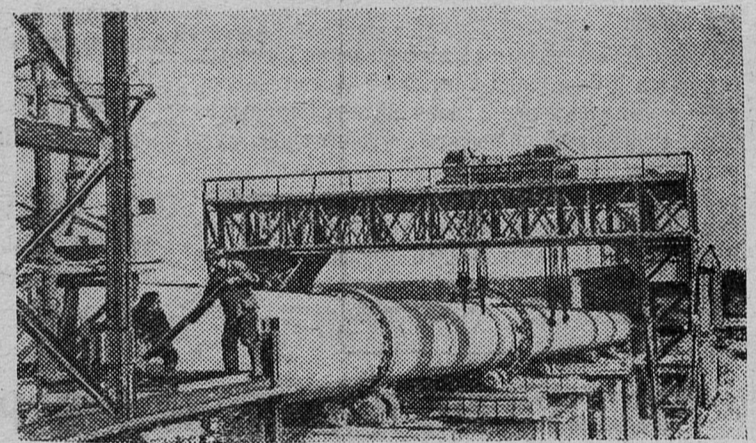
ЛАТВИЙСКАЯ ССР. На Броценском цементно-шиферном комбинате сооружается новая технологическая линия. Заканчивается монтаж 50-метровой вращающейся печи, которая будет производить клинкера значительно больше, чем три действующие.
