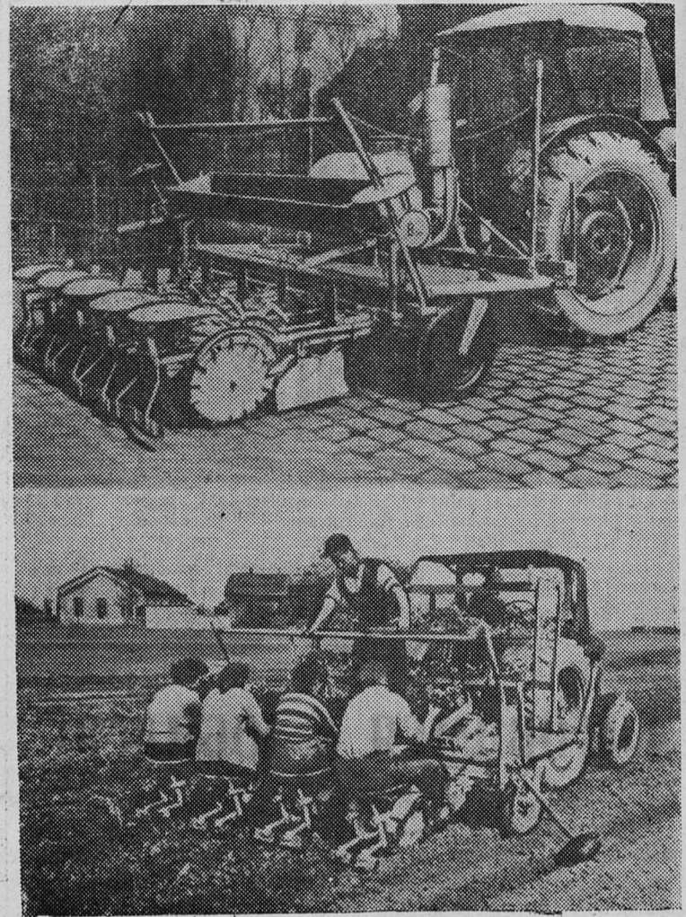
ГЕРМАНСКАЯ ДЕМОКРАТИЧЕСКАЯ РЕСПУБЛИКА. На народном предприятии «Боденбайтунгсерте» в Лейпциге создана новая машина для посадки растений, черенков и картофеля. За час с помощью агрегата может быть высажено от 7 до 10 тысяч растений. Фото Центральбильд—ТАСС
