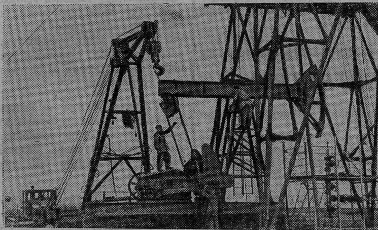
ЧЕЧЕНО-ИНГУШСКАЯ АССР. Участок Гойт-Корт нефтепромыслового управления «Октябрьнефть». С начала года коллектив молодого участка добыл сверх плана около 300 тонн нефти. Для повышения дебита некоторые скважины здесь переводят с фонтанной на глубинно-насосную добычу.
