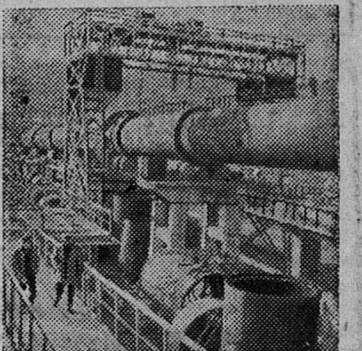
На одной из крупных строек пятилетки — Разданском горно-химическом комбинате в Армянской ССР завершена установка гигантской вращающейся печи цементного завода длиной 185 и диаметром 5 метров.
