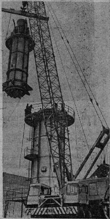
40-метровой высоты достигнет после сборки трубчатая печь для получения бензина, которая будет экспонироваться на весенней международной ярмарке в Лейпциге. Магдебургский завод тяжелого машиностроения имени Карла Либкнехта (ГДР) отправит в этом году пять таких установок в Советский Союз.
