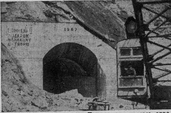
метров воды в секунду. Тоннели полностью отведут воды покоренной горной реки. НА СНИМКАХ: слева — буровзрывные работы на площадке будущего здания ГЭС, справа — входной портал второго тоннеля.
