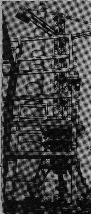
Полным ходом идет реконструкция Среднеуральской ГРЭС, мощность которой достигнет 1 миллиона 372 тысяч киловатт. На снимке: строительство главного корпуса второй очереди.
