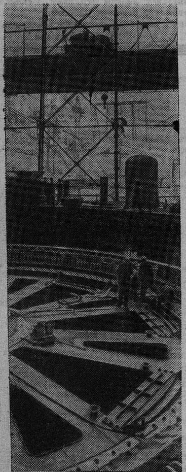
ДИВНОГОРСК. Готовятся к пуску первые два агрегата гигантской гидроэлектростанции на Енисее Красноярской ГЭС. НА СНИМКЕ: монтажные работы на втором агрегате. Фото Ю. Бармина. Фотохроника ТАСС.
