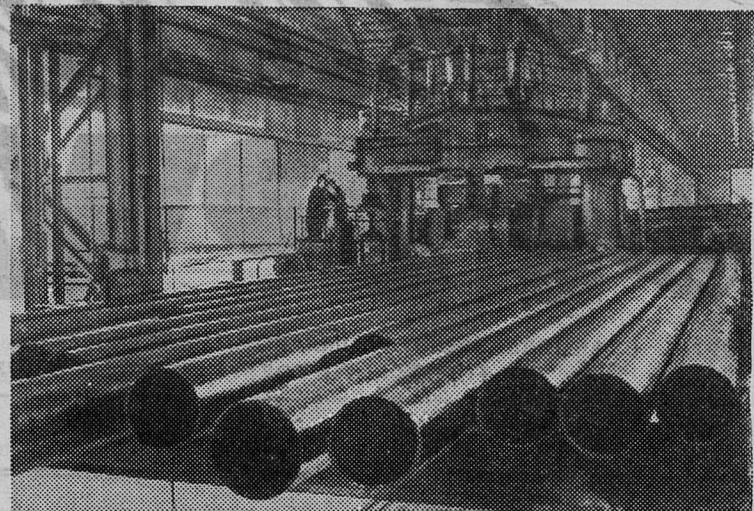
Коллектив Челябинского трубопрокатного завода начал промышленное освоение нового стана холодной прокатки труб — «250». Он будет производить трубы диаметром 100—250 мм высокой прочности, с зеркальной наружной и внутренней поверхностью.
