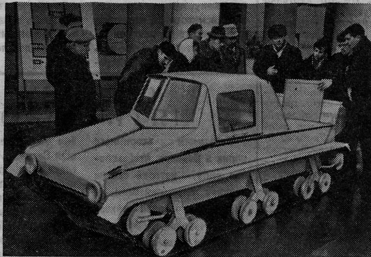
МОСКВА. Этот гусеничный вездеход на воздушной подушке, созданный коллективом Казанского завода имени С. П. Горбунова, можно увидеть сейчас на Выставке достижений народного хозяйства СССР. Благодаря воздушной подушке, уменьшающей его вес на 60—80 процентов, он легко преодолевает заболоченные, заснеженные, песчаные участки пути и водоемы глубиной до 30 сантиметров. Вездеход рассчитан на 2-х человек и 50 килограммов груза. Максимальная скорость 30—40 километров в час. Фото Н. Кулешова. Фотохроника ТАСС
