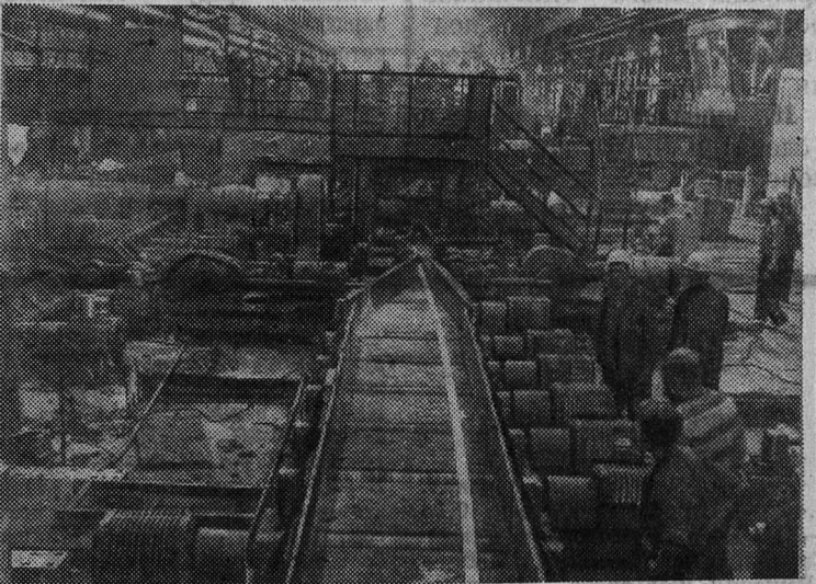
Первый прокат получен на Кировском заводе со стана «350». Новейший, полностью механизированный и автоматизированный агрегат, длиной почти в полкилометра, пришел на смену шести старым сортовым станам, которые демонтированы. Прокатный гигант будет давать вдвое больше продукции, а для обслуживания его потребуется вдвое меньше рабочих.
