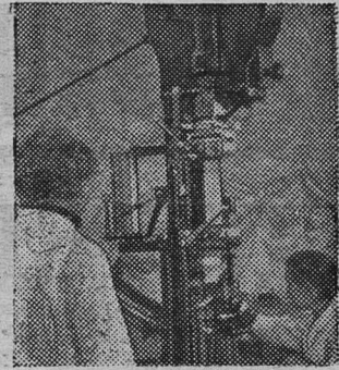
Испытание ткани на разрыв для парашюта спускаемого аппарата автоматической межпланетной станции «Венера-7». (Кадр из цветного научно-популярного фильма «К планете загадок». Фотохроника ТАСС)
