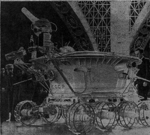
Москва. Экспозиция павильона «Космос» Выставки достижений народного хозяйства СССР пополнилась новым уникальным экспонатом. Здесь установлена точная копия первой передвижной автоматической лаборатории «Луноход-1» для комплексного изучения особенностей строения лунной поверхности, окололунной среды и дальних космических объектов. Фото Н. Хренникова (Фотохроника ТАСС)
