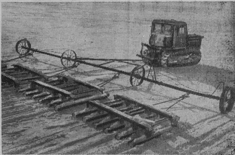
УЛЬЯНОВСКАЯ ОБЛАСТЬ. Снегозадержание ведут механизаторы совхоза имени Н. К. Крупской Мелекесского района. На полях, занятых посевами озимых, эту работу производят с помощью специальных агрегатов, изготовленных рационализаторами хозяйства. Своеобразные снегопахи дают возможность накапливать влагу даже при неглубоком снежном покрове.
