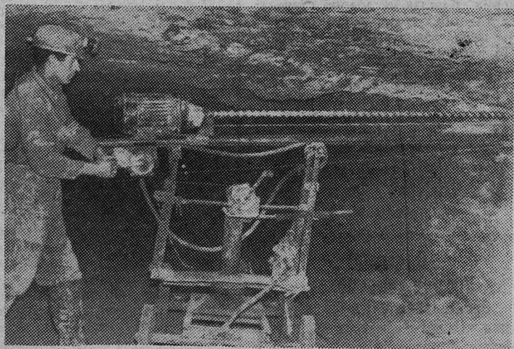
НА СНИМКЕ: горнорабочий при помощи бурильного станка бурит шпур.
