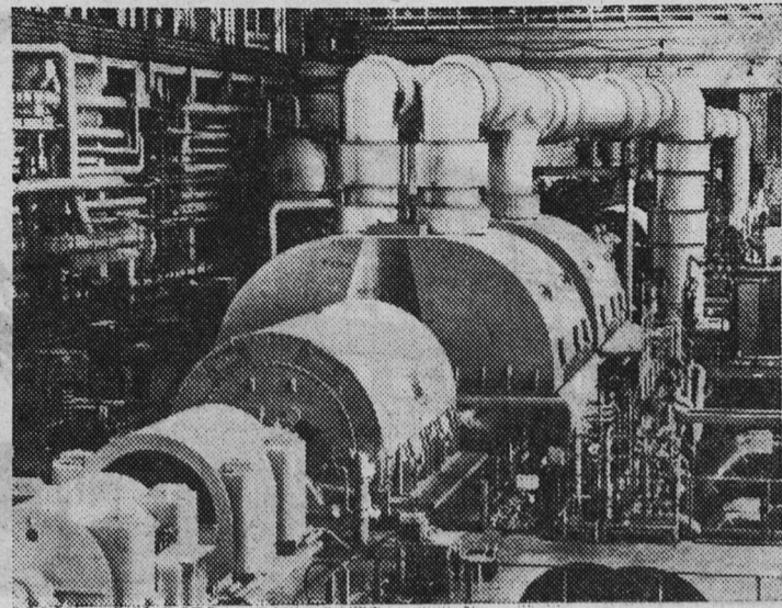
Турбинный зал атомной электростанции, сооружаемой близ Грейфсвальда на севере Германской Демократической Республики. Недавно здесь дал ток первый энергоблок мощностью 440 тысяч киловатт. Создание современной крупной АЭС — результат социалистической экономической интеграции. Участники «стройки дружбы» — Советский Союз, Венгрия, Польша, Чехословакия. Фото АДН—ТАСС
