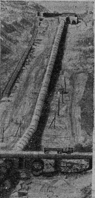
НА СНИМКЕ: участок Томуловского дюкера. Этот трубопровод собран из колец диаметром 4 метра.
